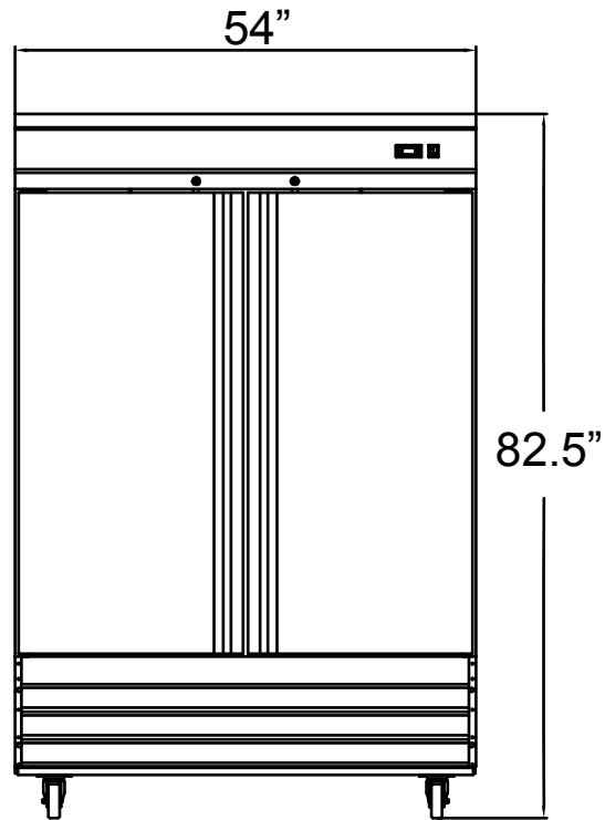
ELEVATION
